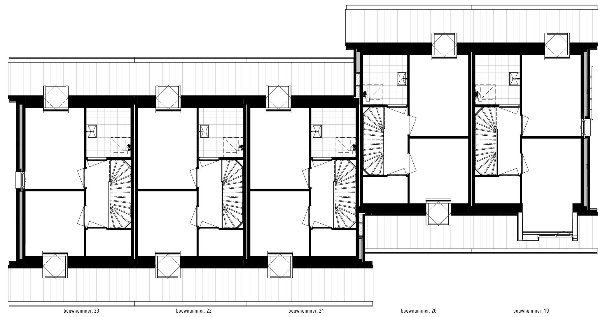
1ste verdieping
