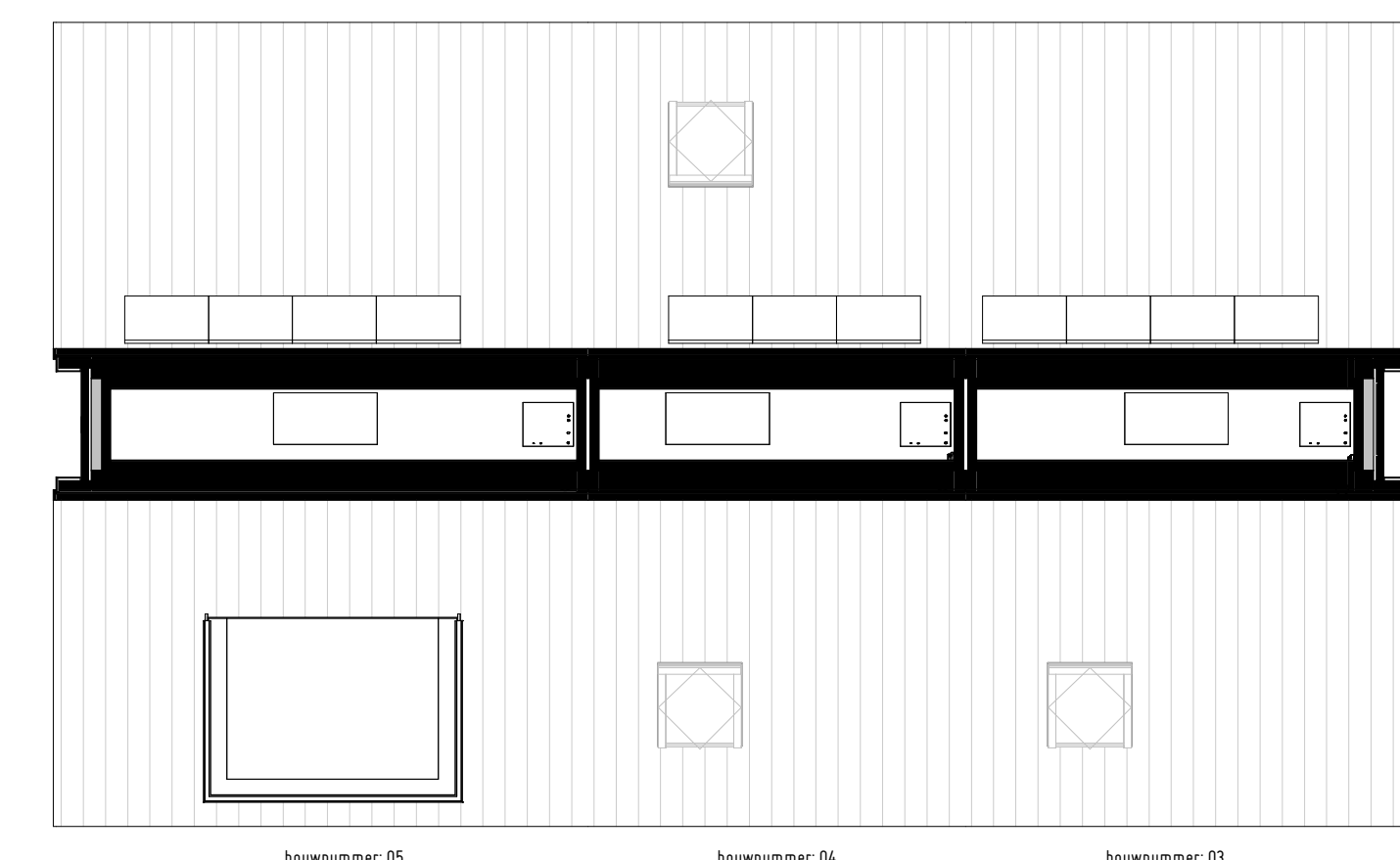
2de verdieping
