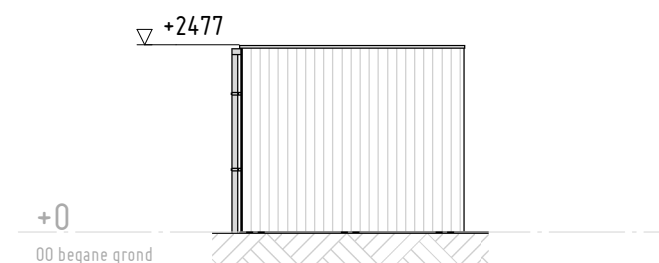
Rechter zijgevel_rij berging
