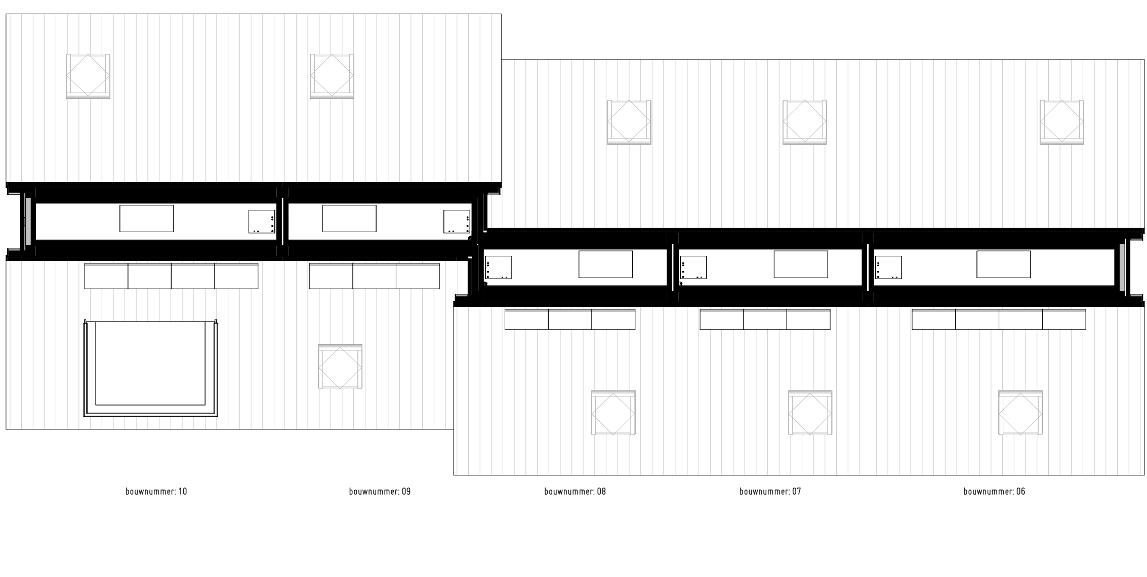
2de verdieping
