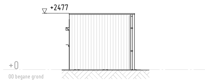
voorgevel_enkele berging
