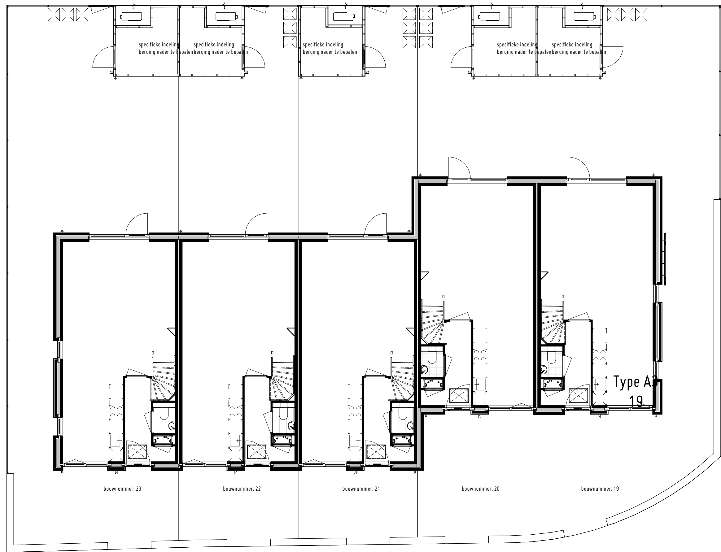
Begane grond
