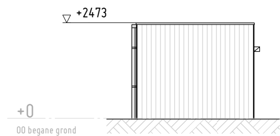
Rechter zijgevel_enkele berging
