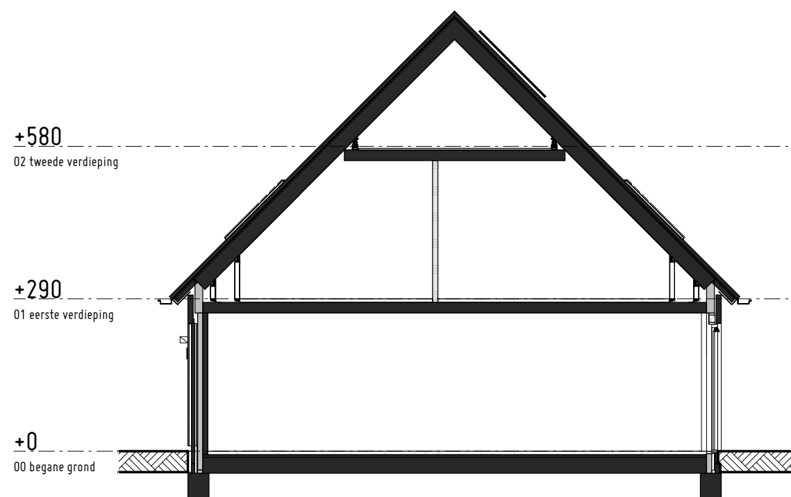
Doorsnede
