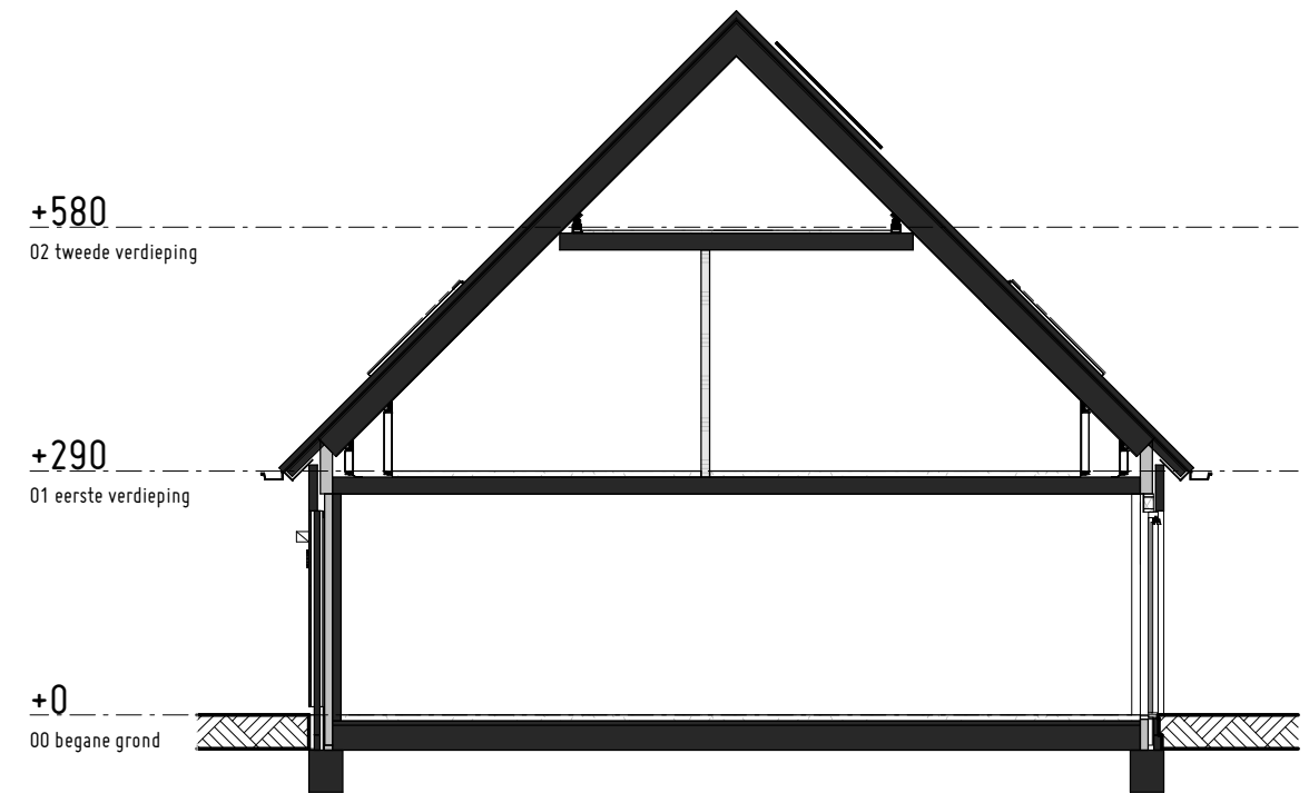
Doorsnede
