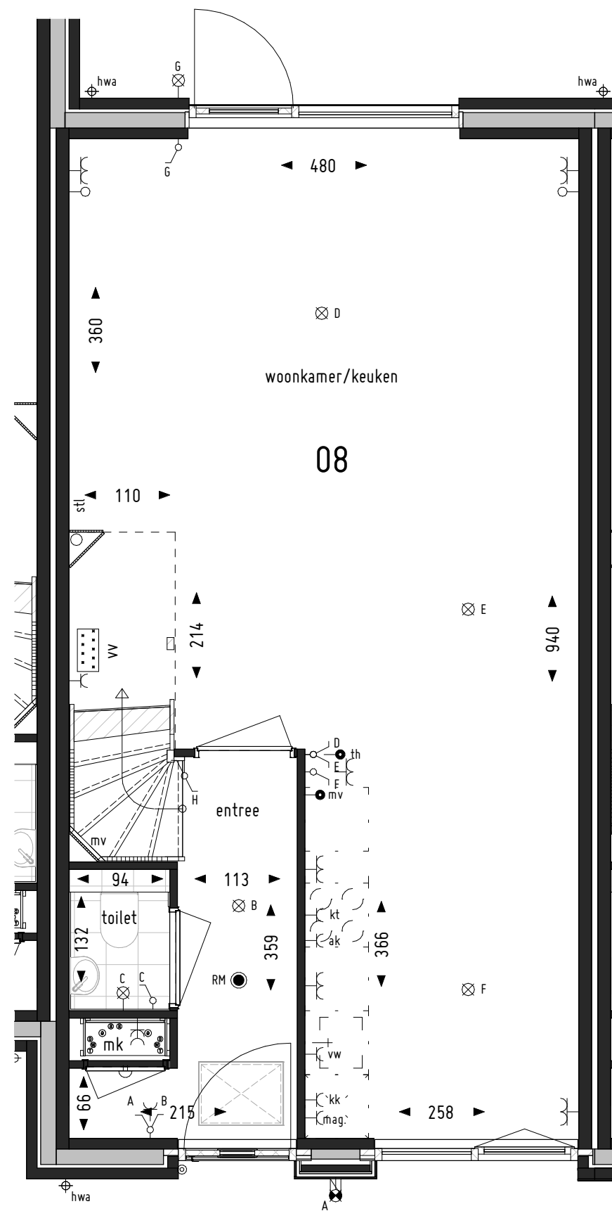
Begane grond
