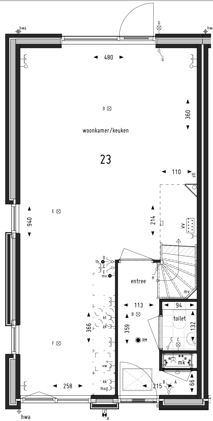
Begane grond
