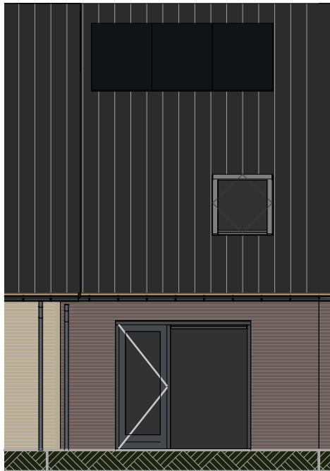
bouwnummer: 21 Achtergevel
