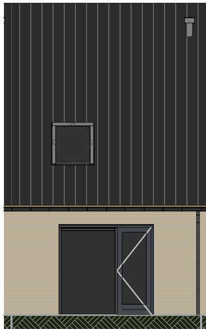
bouwnummer: 07 Achtergevel
