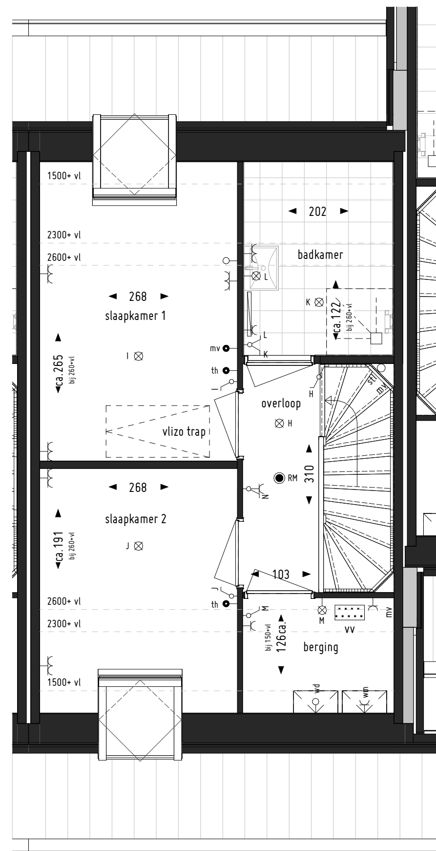
1ste verdieping
