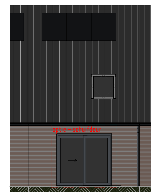
Achtergevel bouwnummers; 4, 7, 8, 9, 19, 20, 21, 22 & 23
