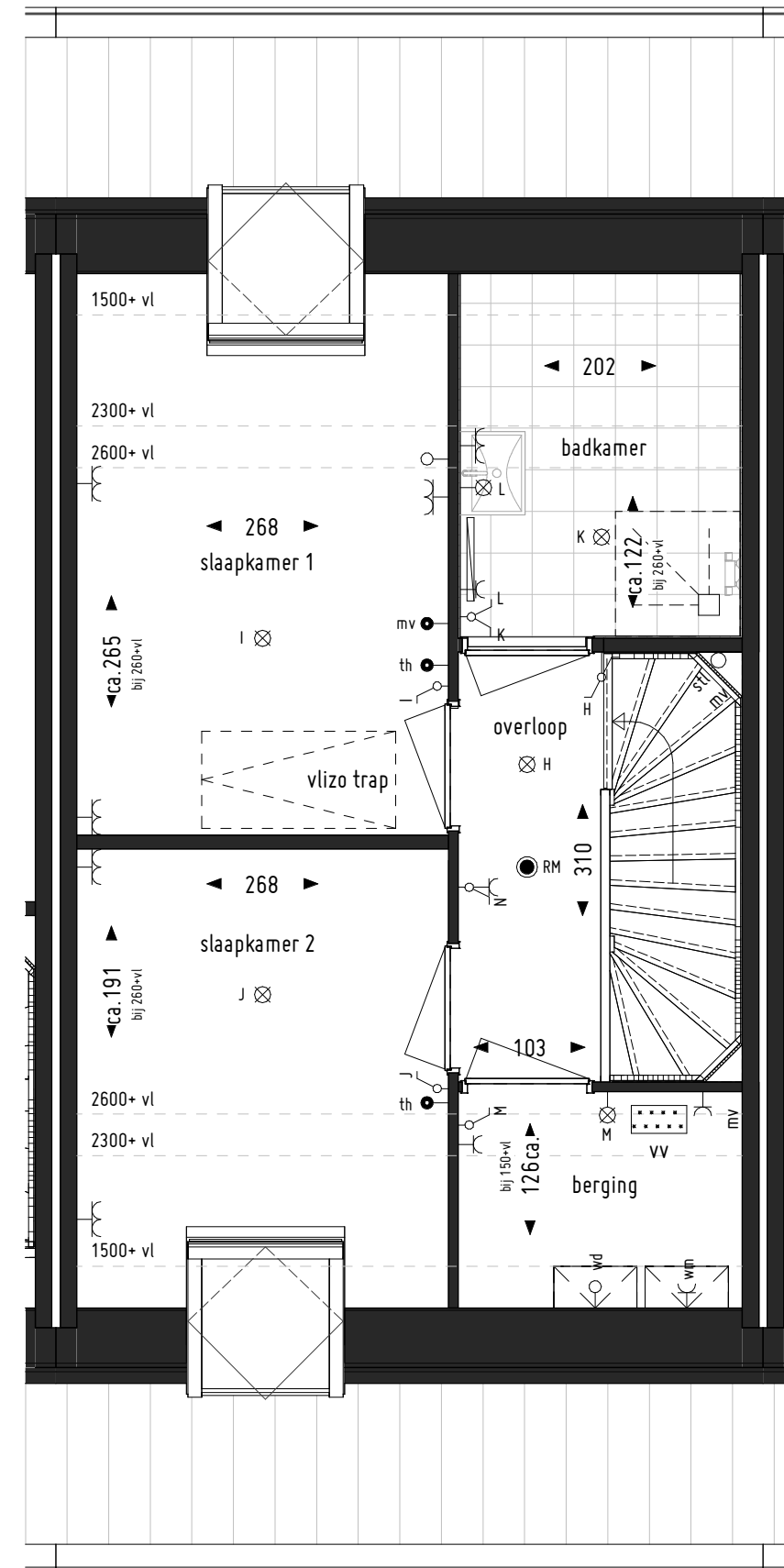
1ste verdieping
