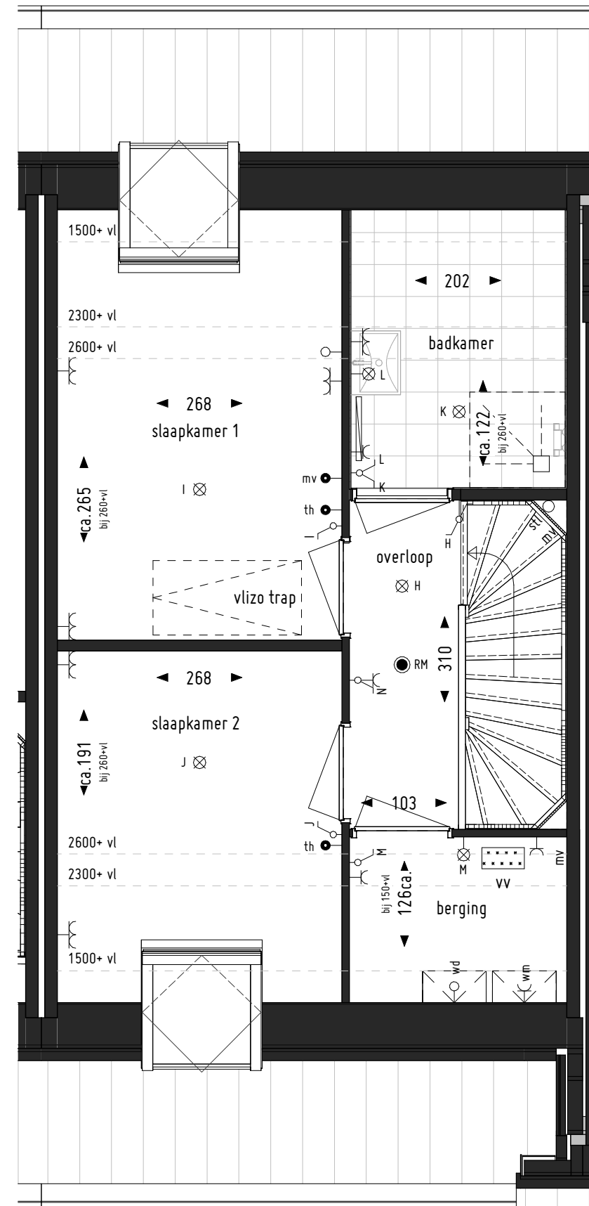
1ste verdieping
