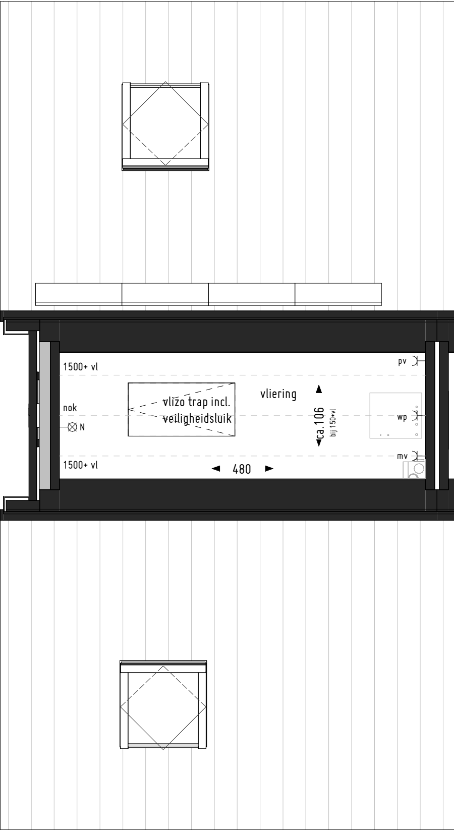
2de verdieping
