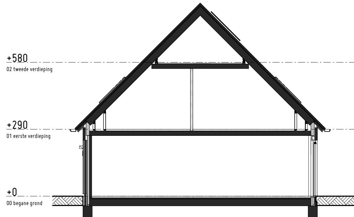
Doorsnede
