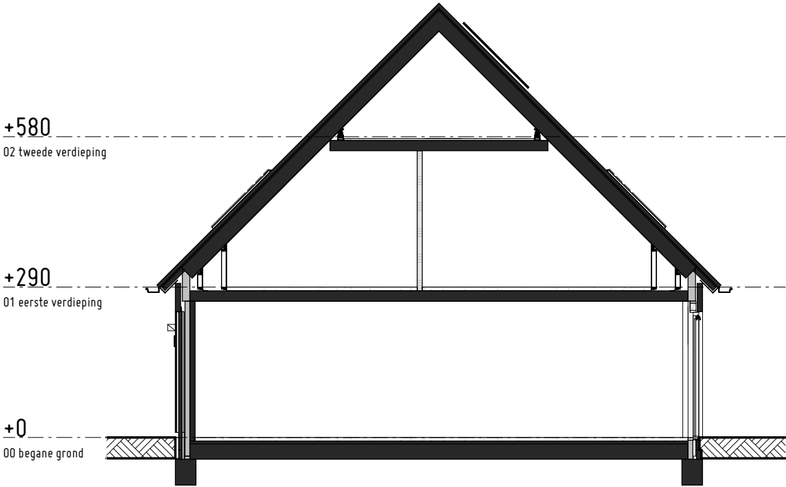
Doorsnede
