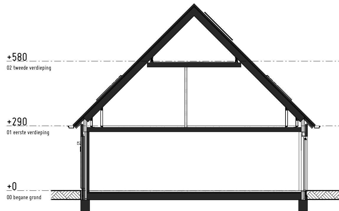
Doorsnede
