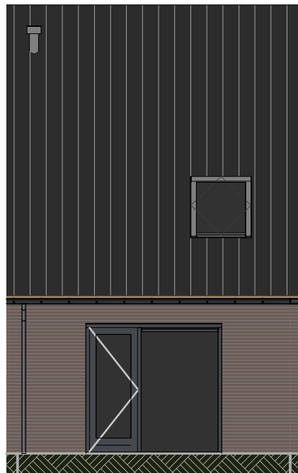
bouwnummer: 09 Achtergevel
