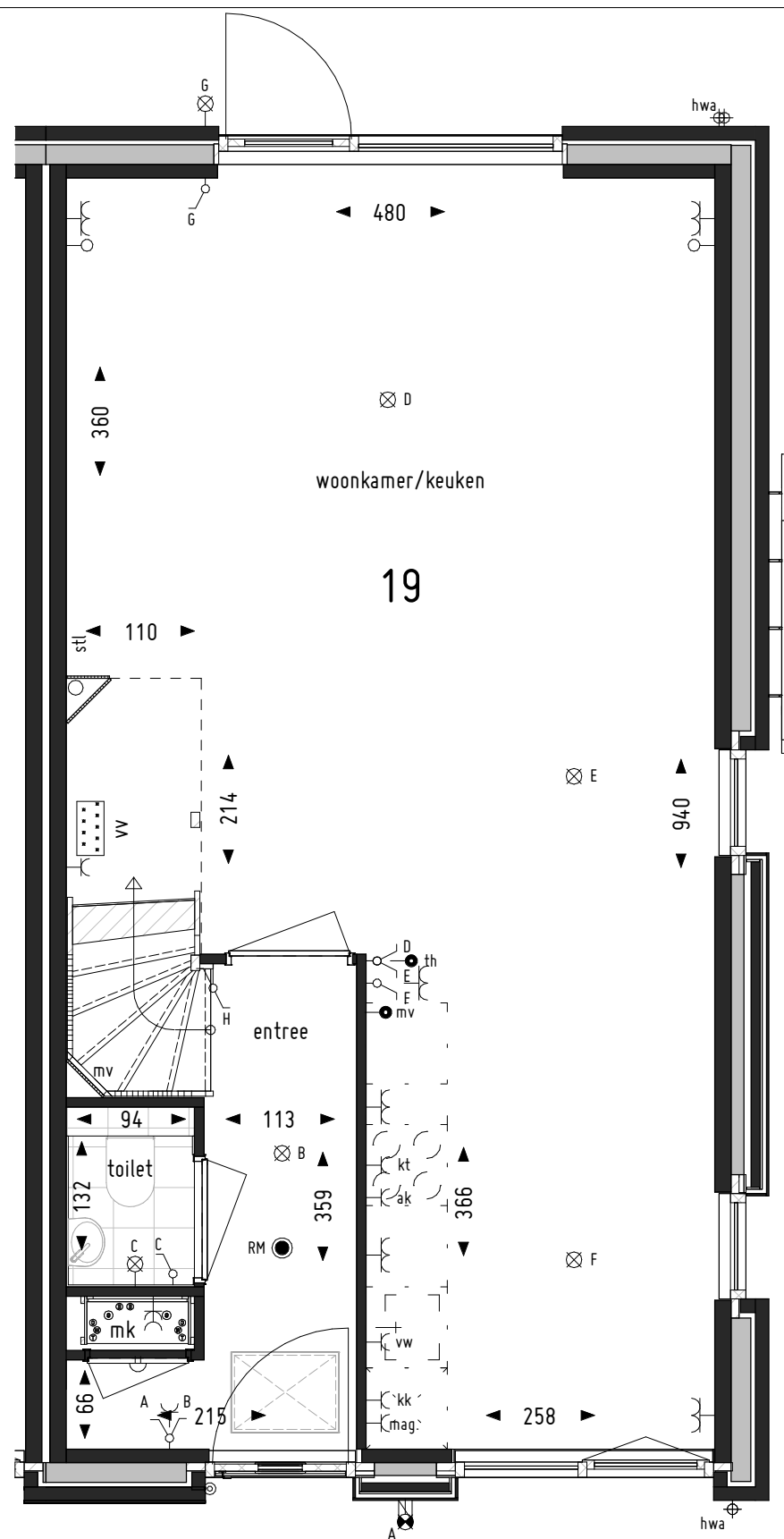
Begane grond
