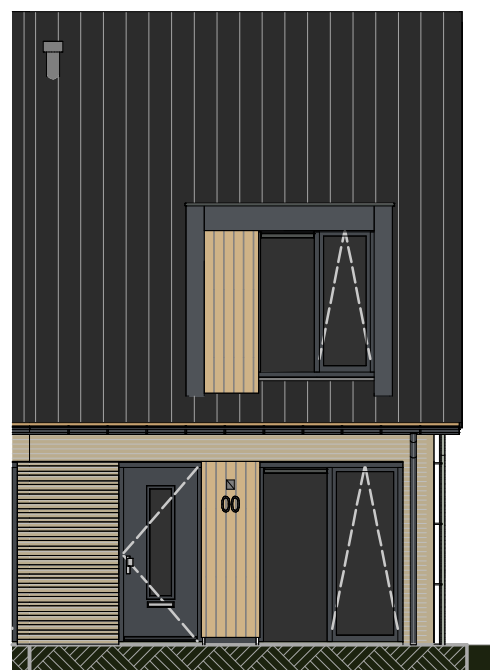
bouwnummer: 19 Vorgevel
