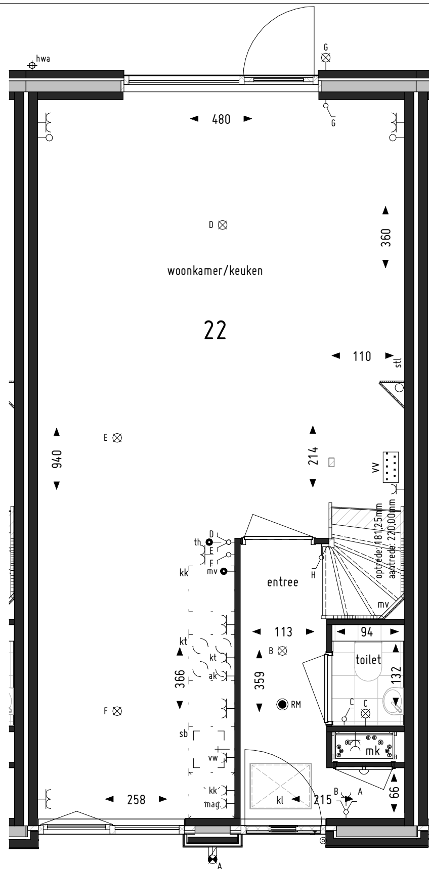
Begane grond
