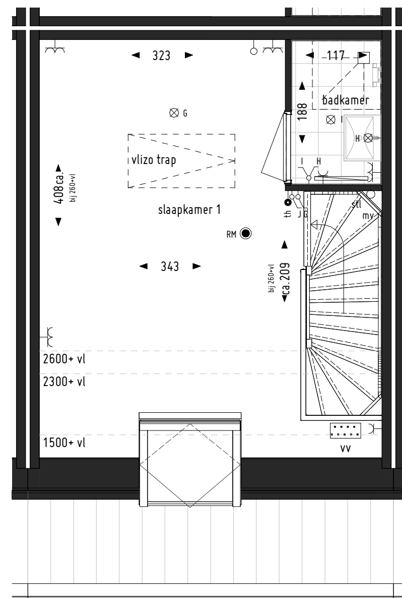
1ste verdieping
