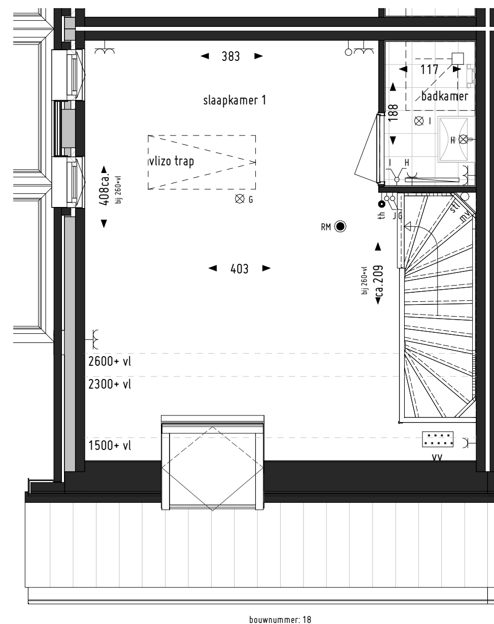
1ste verdieping
