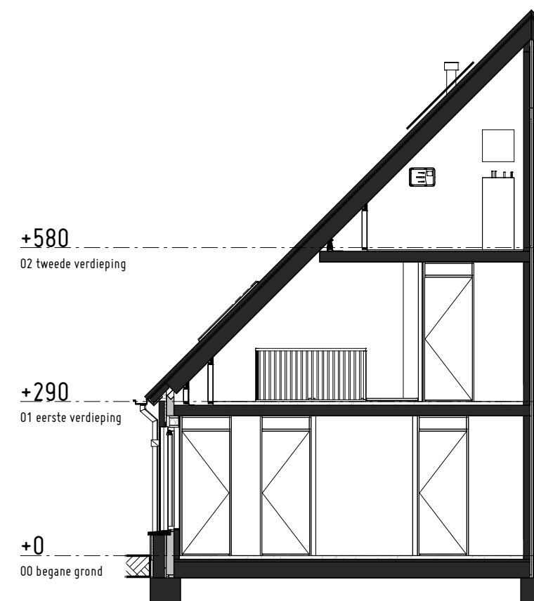
Doorsnede
