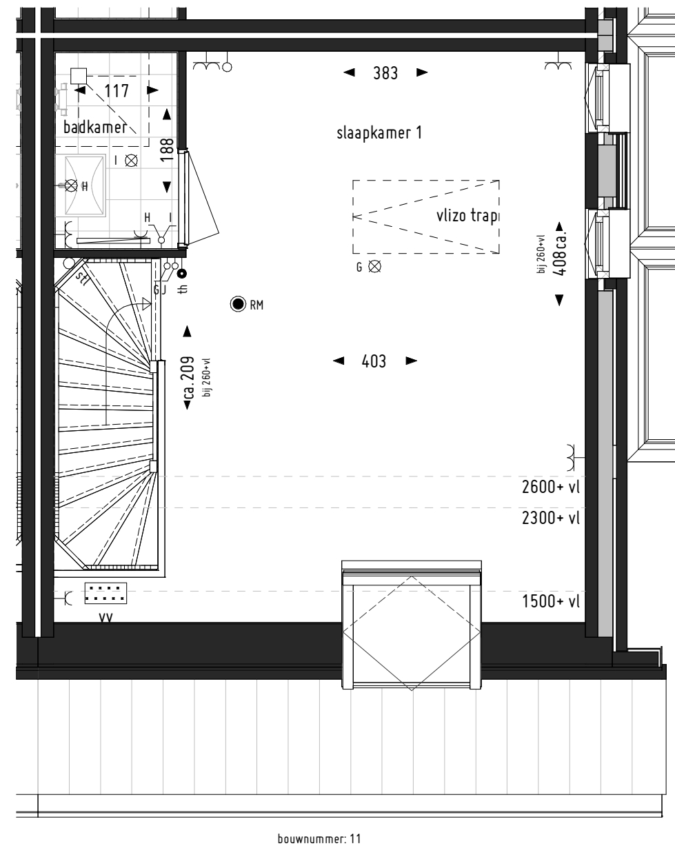
1ste verdieping
