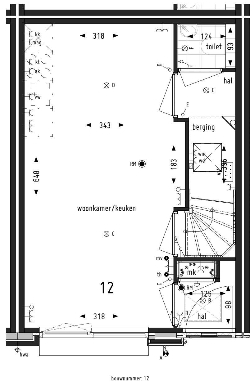
Begane grond
