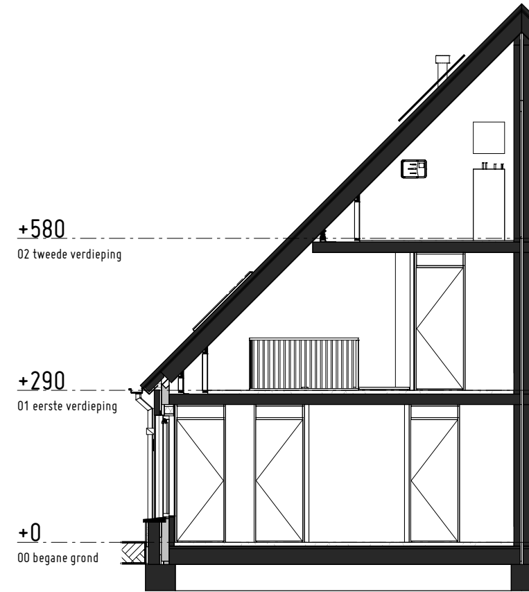
Doorsnede
