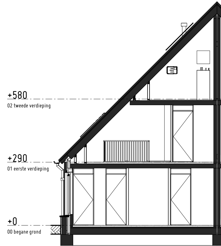
Doorsnede
