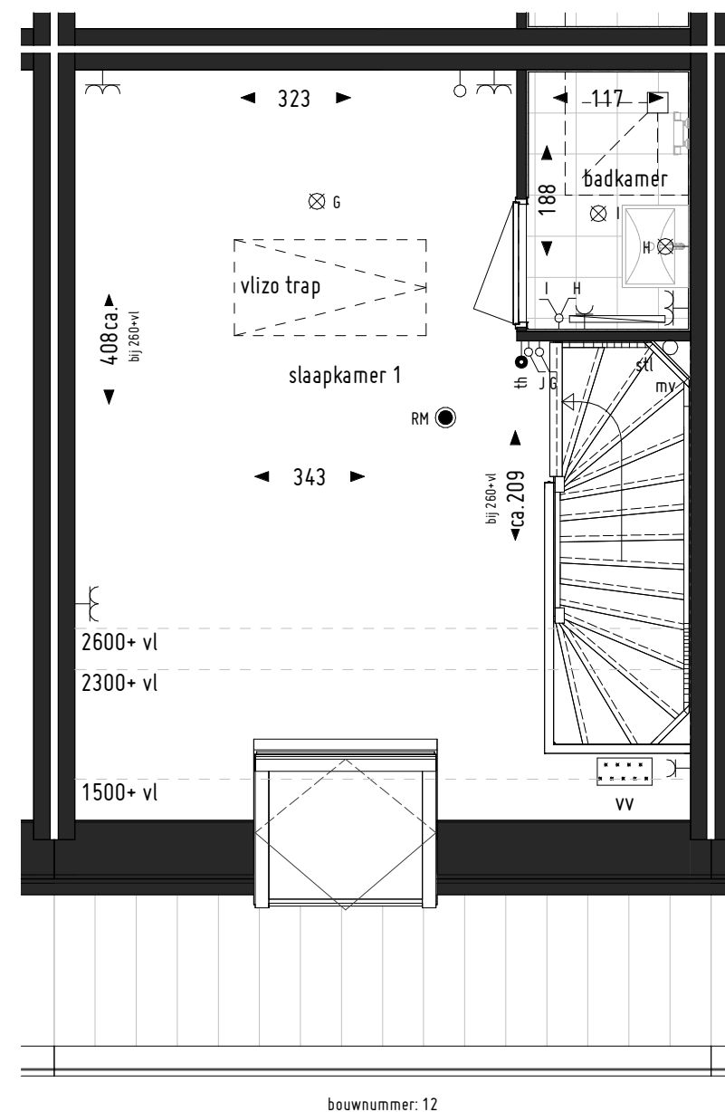
1ste verdieping
