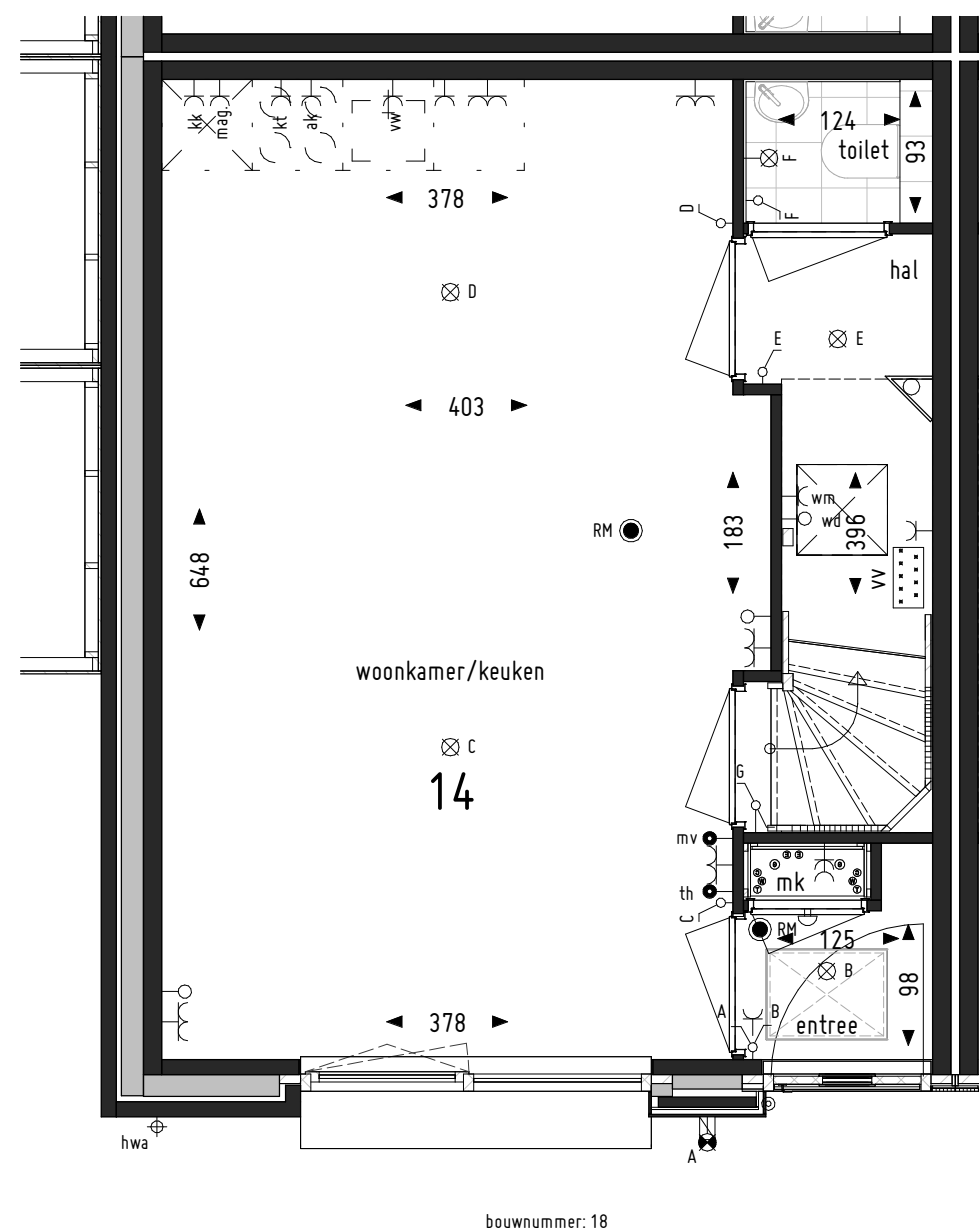
Begane grond
