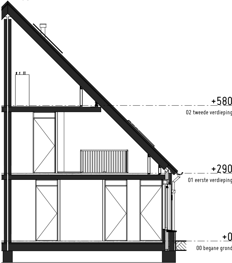
Doorsnede
