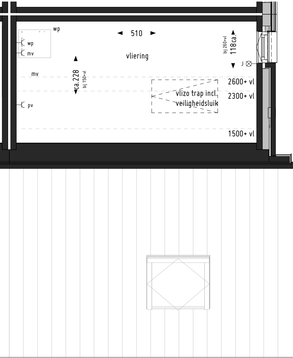
2de verdieping
