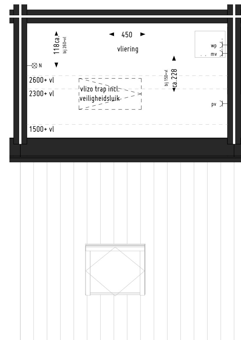
2de verdieping
