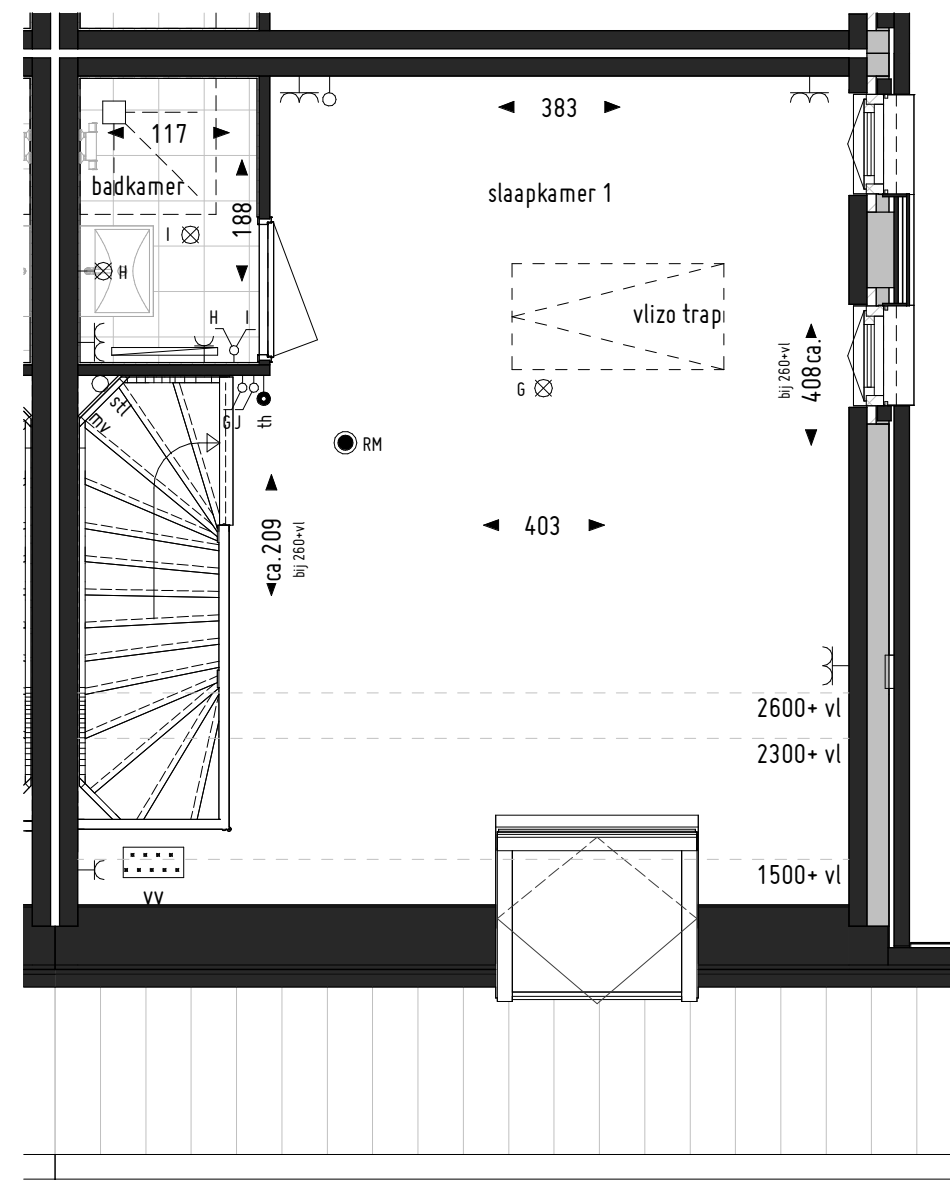
1ste verdieping
