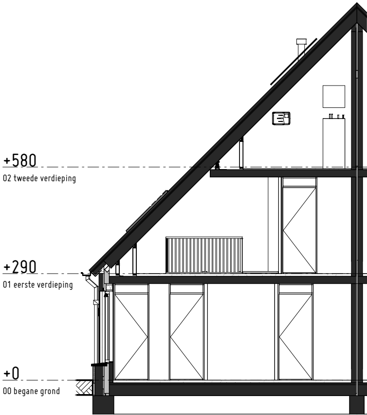
Doorsnede
