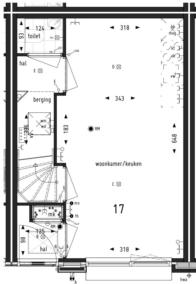
Begane grond
