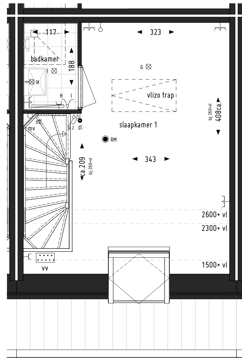
1ste verdieping
