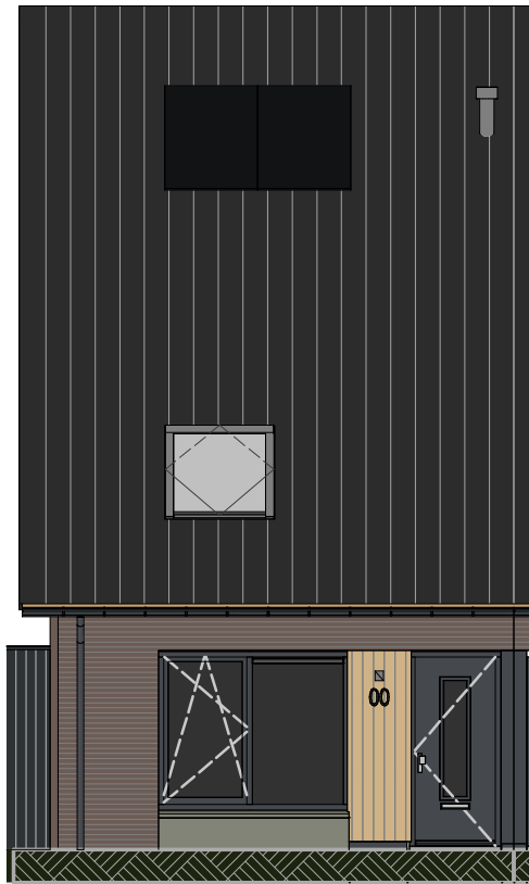
Achtergevel bouwnummer: 18
