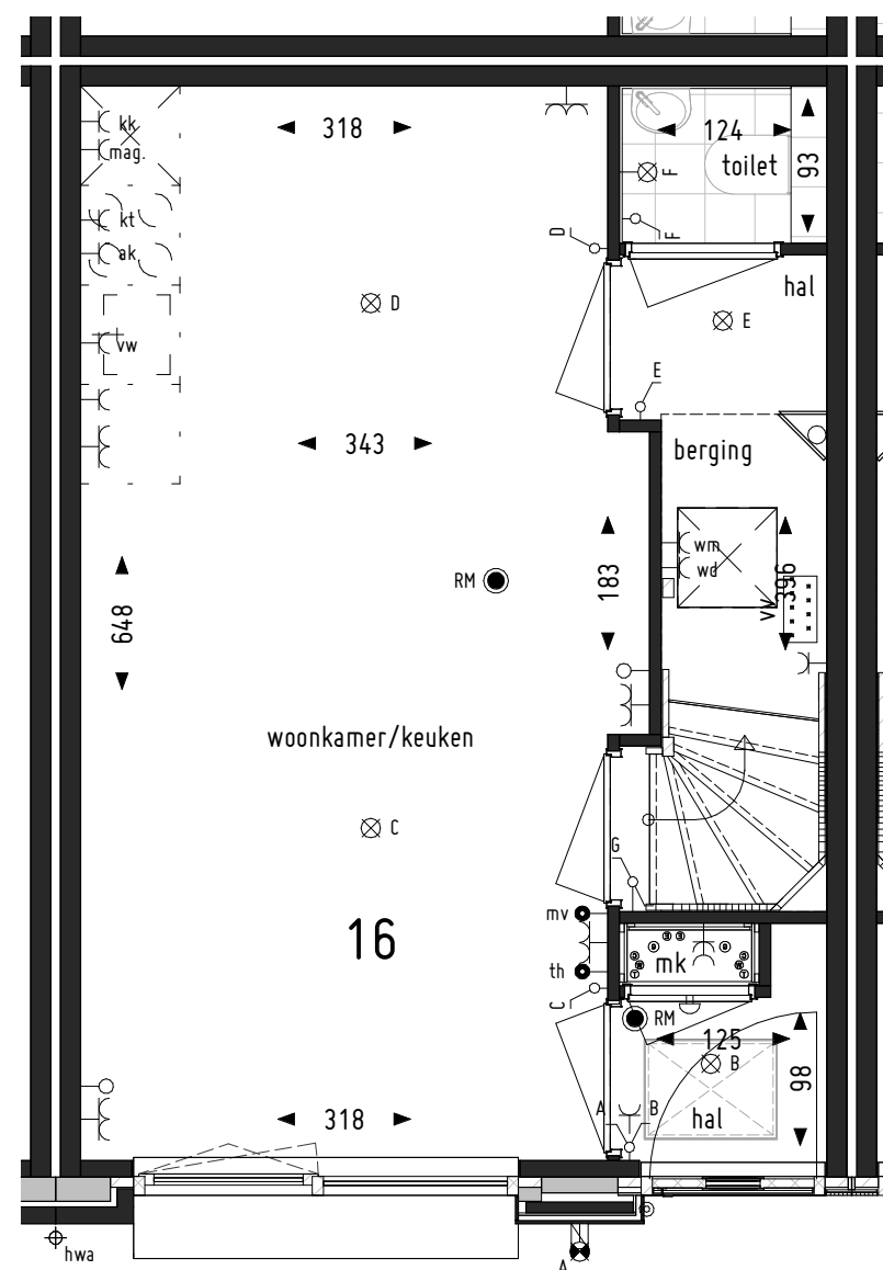
Begane grond
