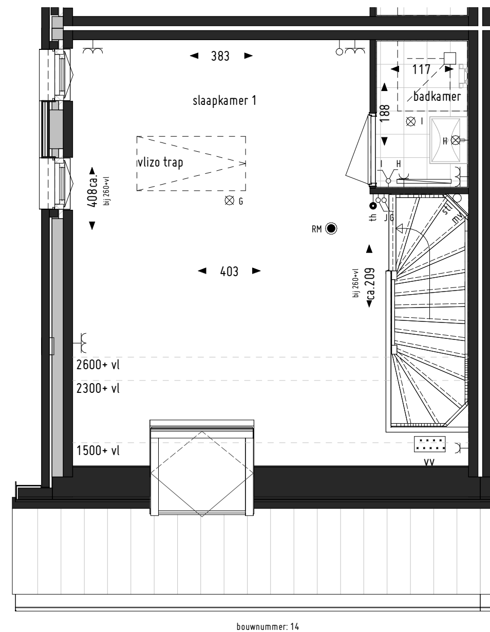
1ste verdieping
